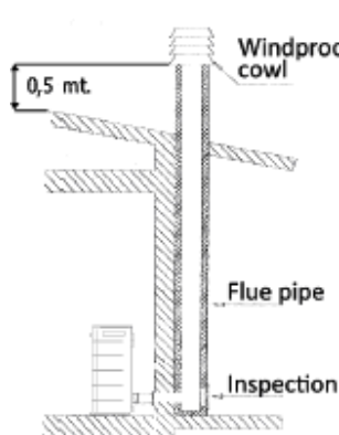
Rys. 2 podłączenie do przewodu spalinowego
