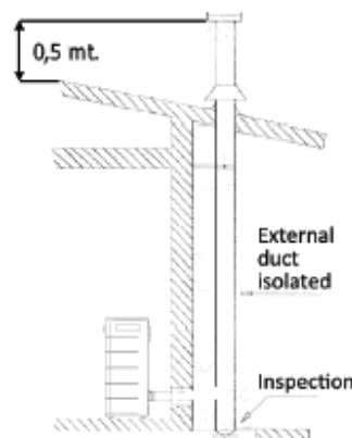
Rys. 3 podłączenie do zewnętrznego izolowanego przewodu spalinowego
