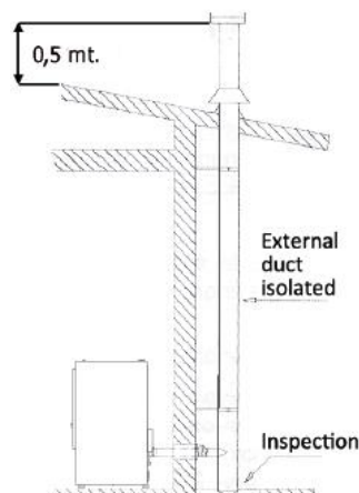
Rys. 3 podłączenie do zewnętrznego izolowanego przewodu spalinowego
